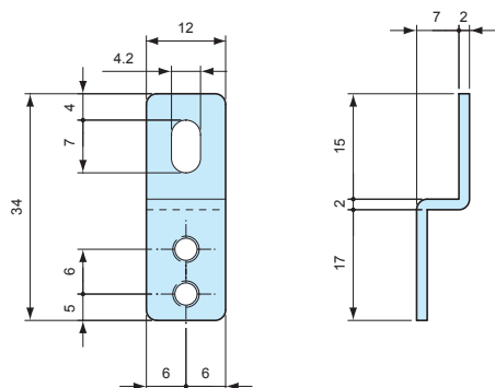
CK-34Z dimensions
