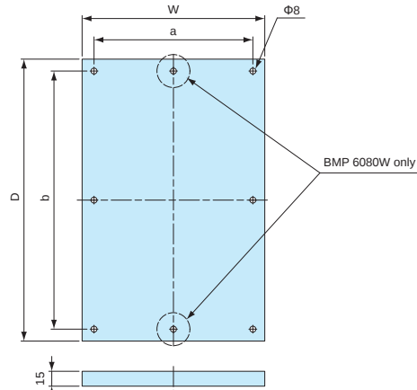
BMP5060W ~ 6080W
