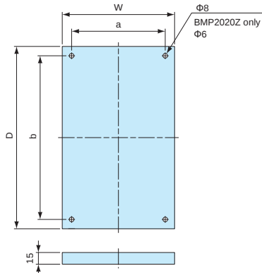
BMP1928W ~ 4060W
