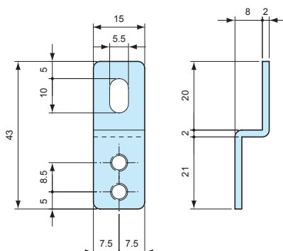
CK-35P dimensions
