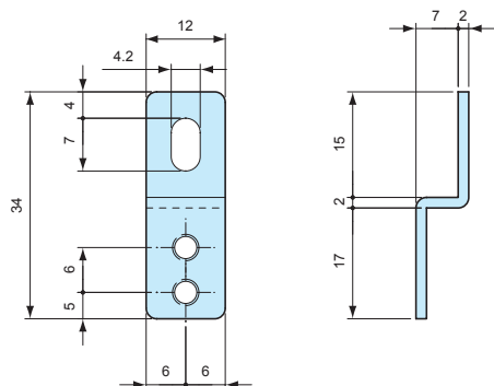
CK-34Z dimensions
