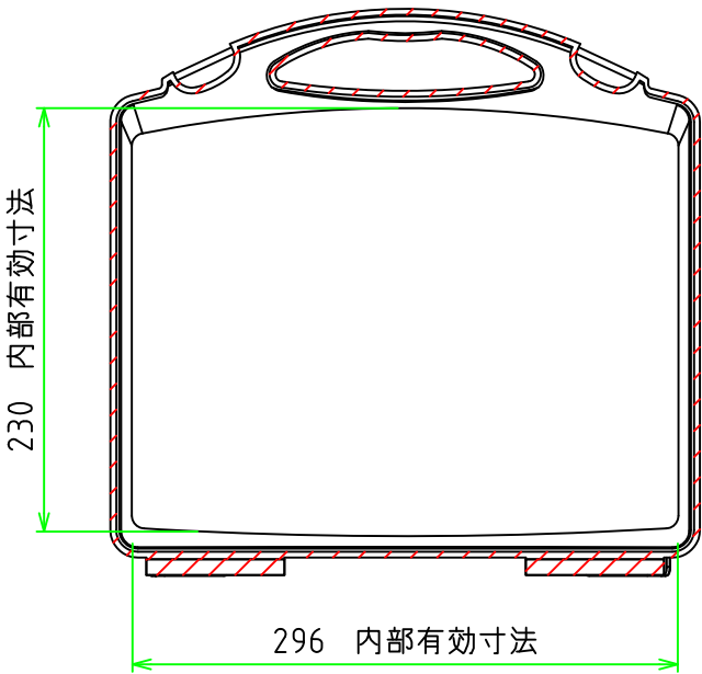
B-B 断面図
