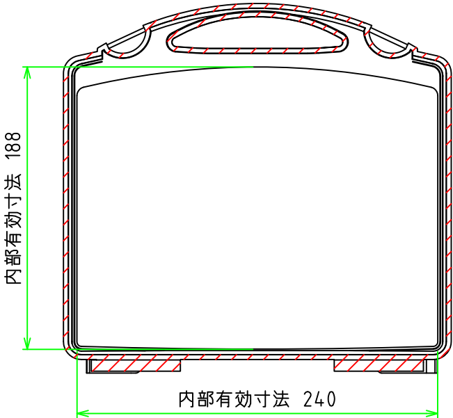
B-B 断面図
