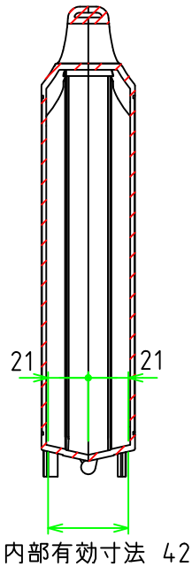
A-A 断面図
