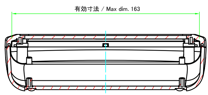
B-B ( 1 : 2 )
