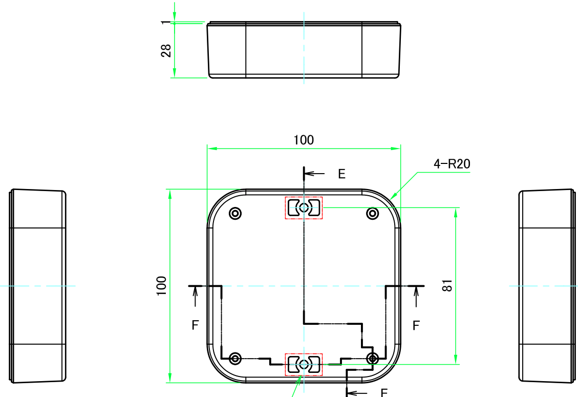
2-ポールマウントブラケット(WPMB-M4)用取付ガイド 2-Mounting position for Pole Mounting Bracket (WPMB-M4)
