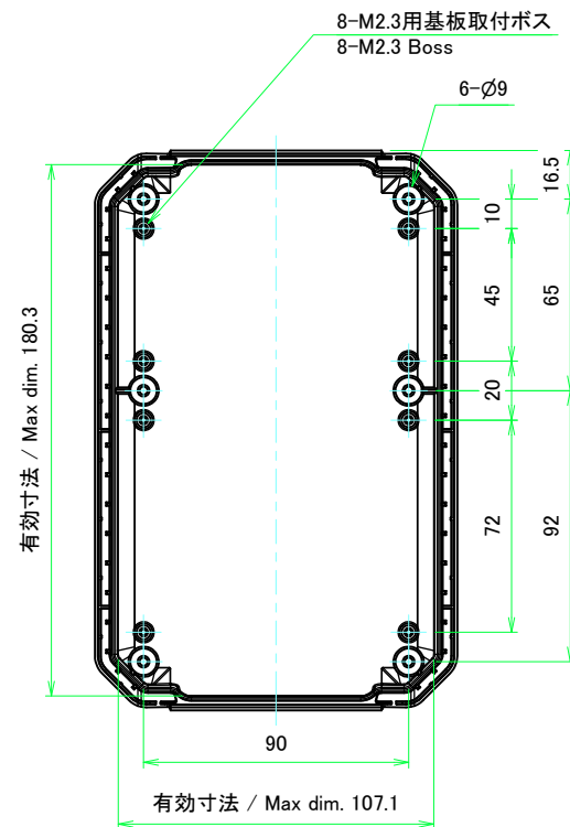
B-B (1:2)
