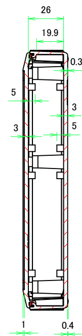
B-B (1:2)
