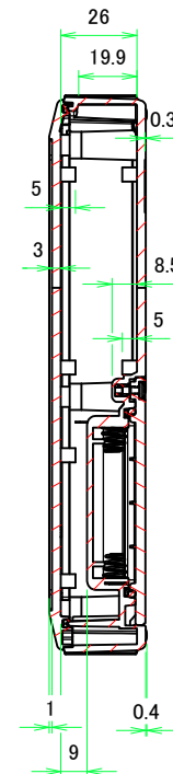
A-A (1:2)
