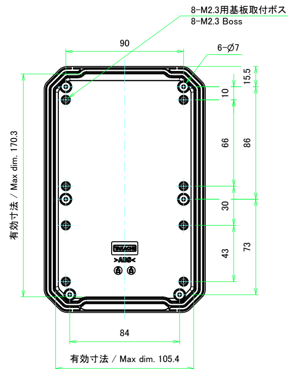
B-B (1:2)
