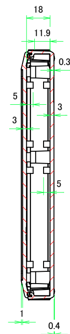
B-B (1:2)
