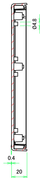
B-B (1:2)
