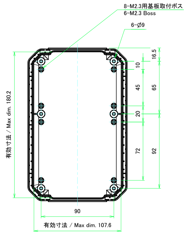
B-B (1:2)
