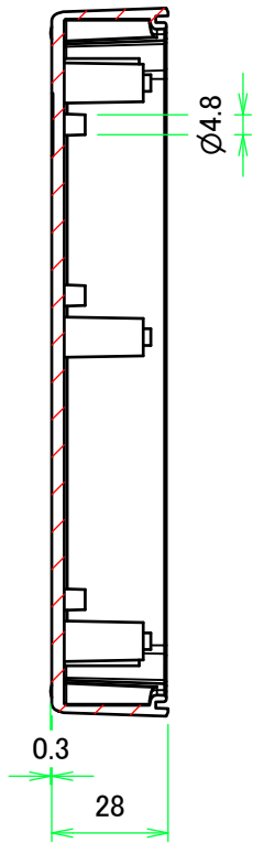
B-B ( 1 : 2 )
