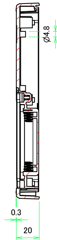
B-B (1:2)
