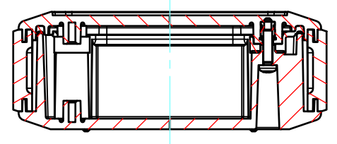
A-A ( 1 : 1.5 )
