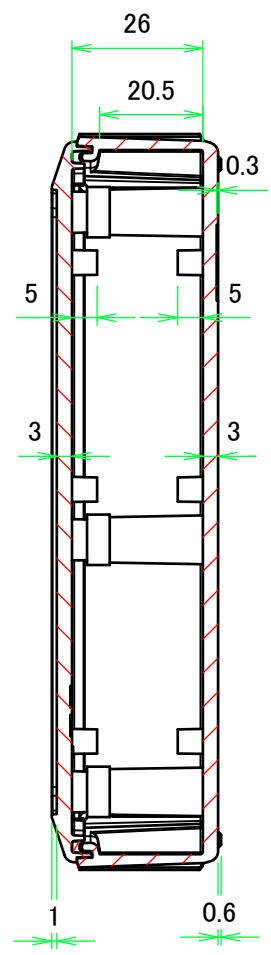
B-B ( 1 : 1.5 )
