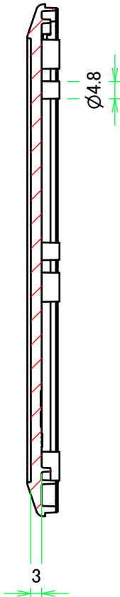
B-B ( 1 : 1.5 )
