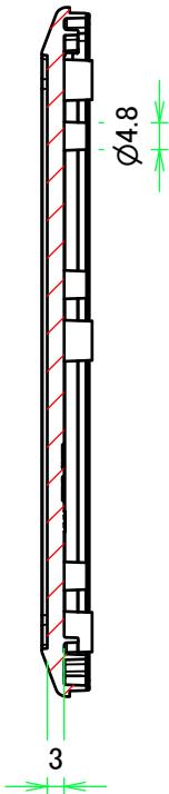
B-B ( 1 : 1.5 )
