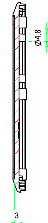
B-B ( 1 : 1.5 )
