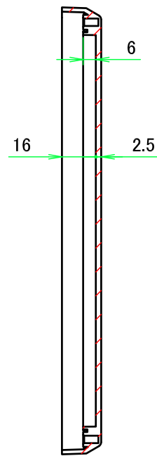
C-C ( 1 : 2.5 )
