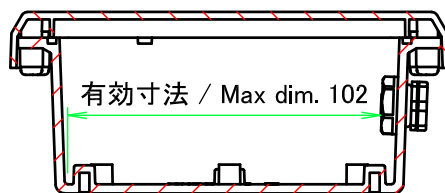
B-B (1:2.5)
