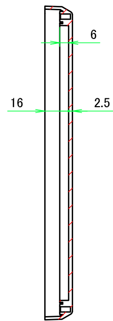
C-C ( 1 : 2.5 )
