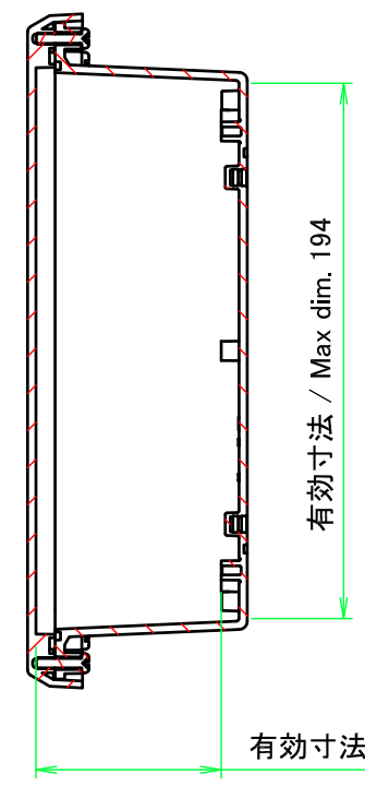
A-A ( 1 : 3 )
