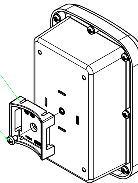
①マウントブラケット Pole mount bracket
