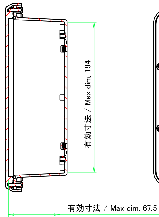
A-A ( 1 : 3 )
