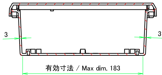
B-B ( 1 : 3 )
