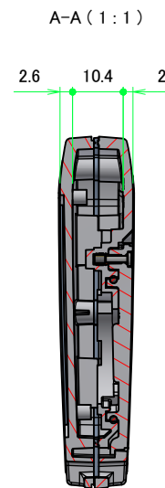
A-A (1:1)
