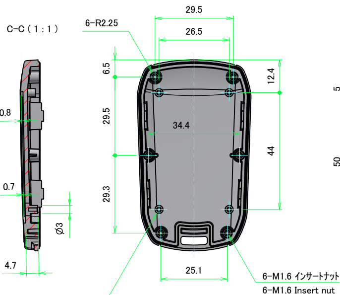
4-M1.6用基板取付ボス 4-M1.6 Boss
