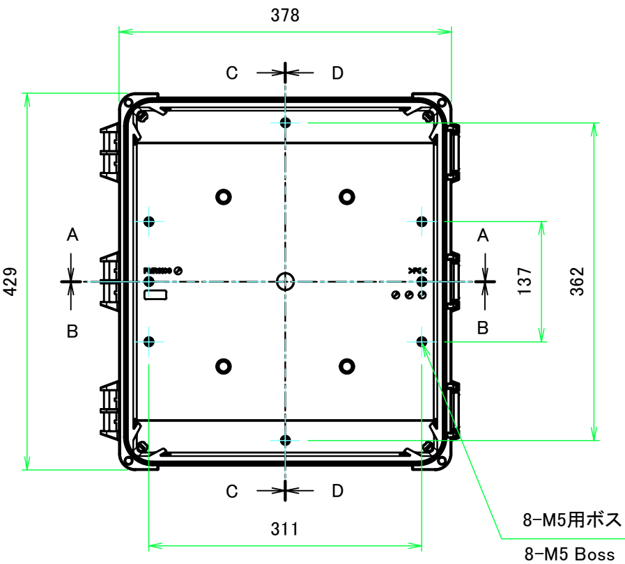
ボディー (内視) Base (Internal View)
