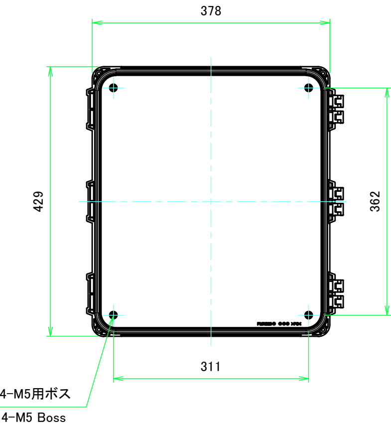
カバー (内視) Cover (Internal View)
