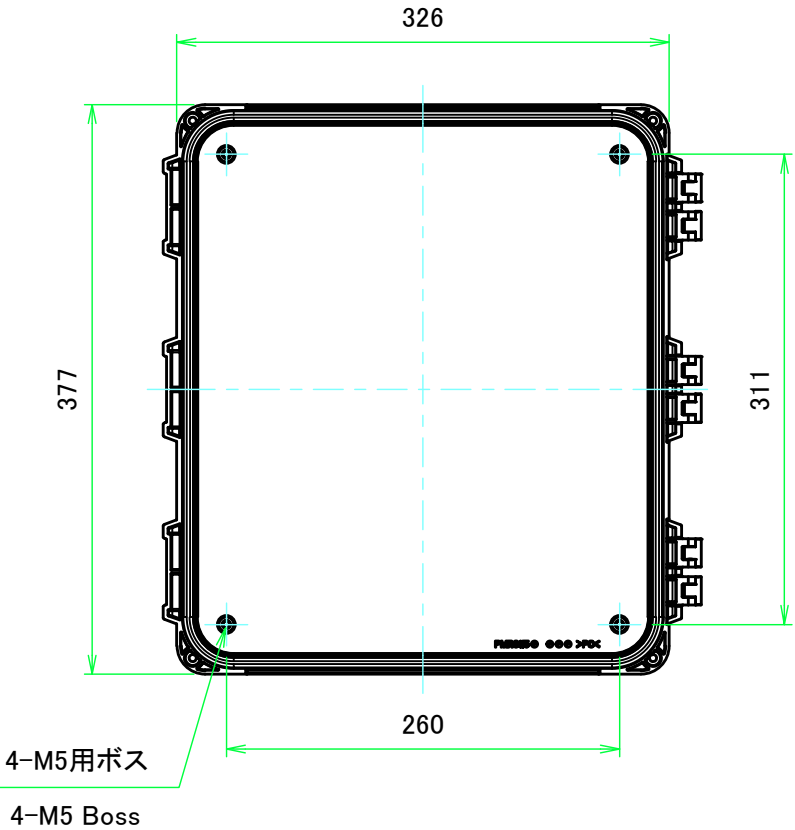
カバー (内視) Cover (Internal View)
