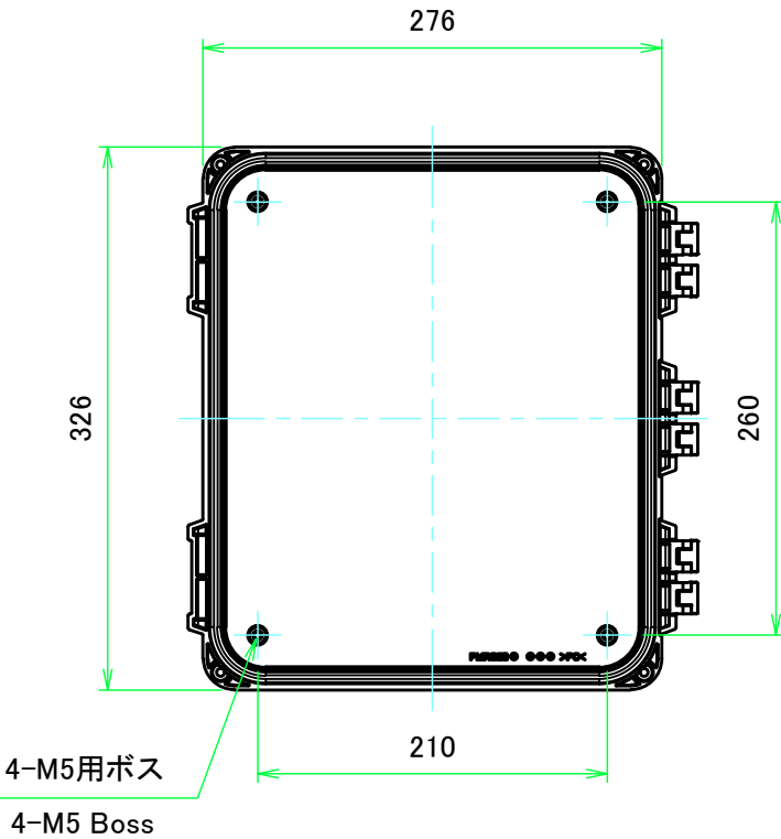
カバー (内視) Cover (Internal View)
