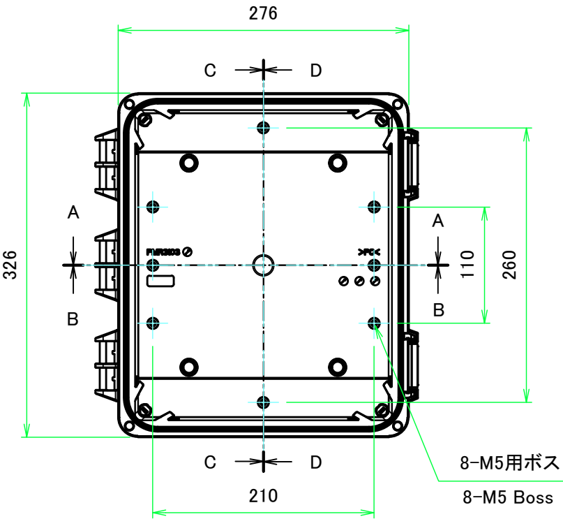
ボディー (内視) Base (Internal View)
