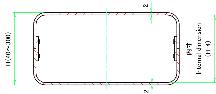
D-D ( 1 : 1.5 )
