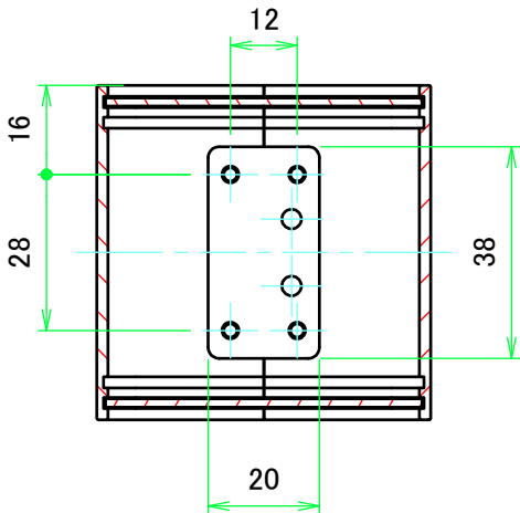
A-A ( 1 : 1.5 )
