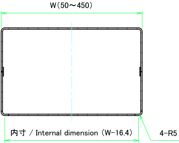
C-C ( 1 : 5 )
