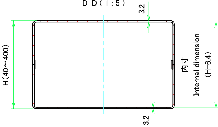
D-D ( 1 : 5 )
