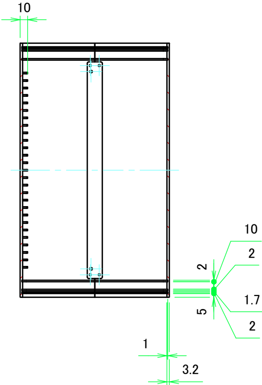
B-B ( 1 : 5 )
