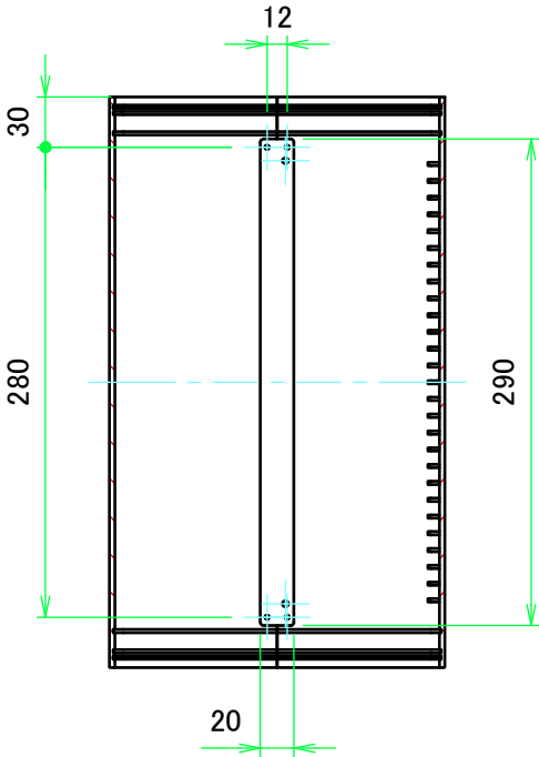
A-A ( 1 : 5 )
