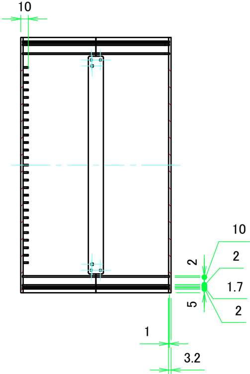
B-B ( 1 : 5 )
