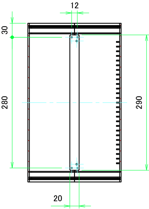
A-A ( 1 : 5 )
