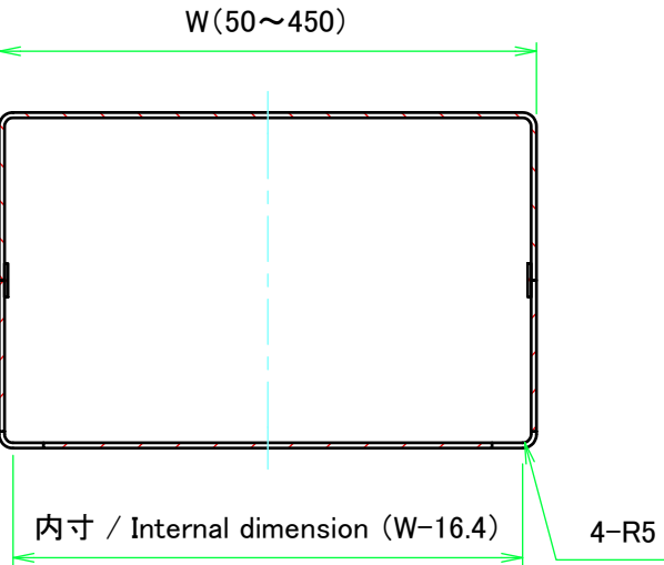
C-C ( 1 : 5 )
