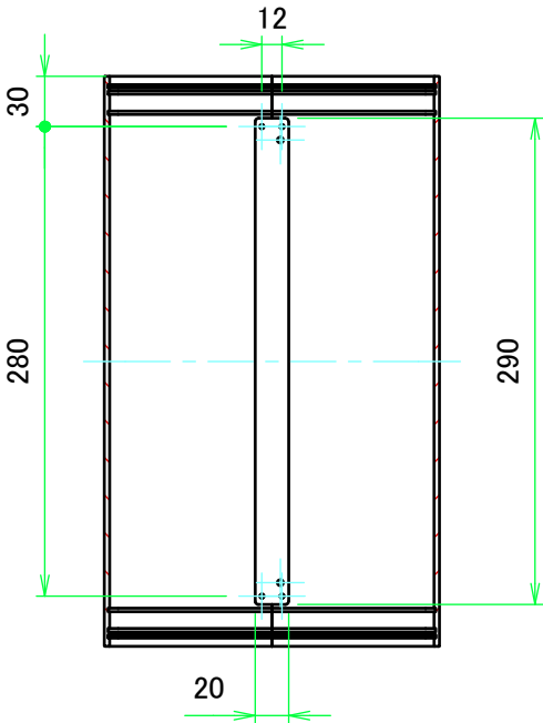
A-A ( 1 : 5 )
