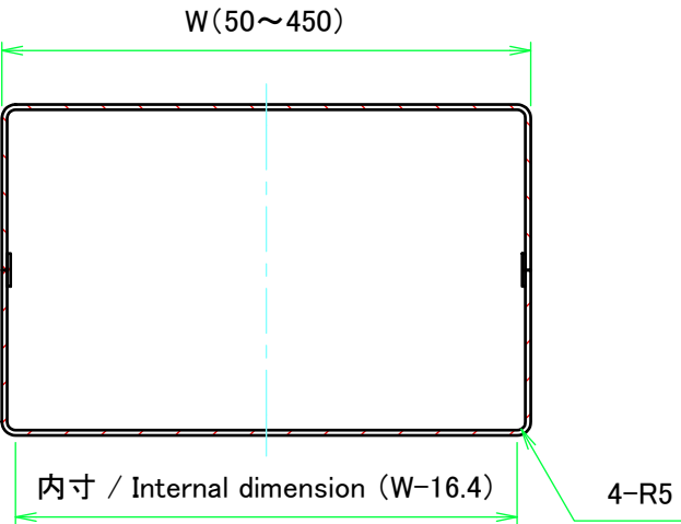
C-C ( 1 : 5 )
