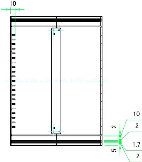
B-B ( 1 : 4 )
