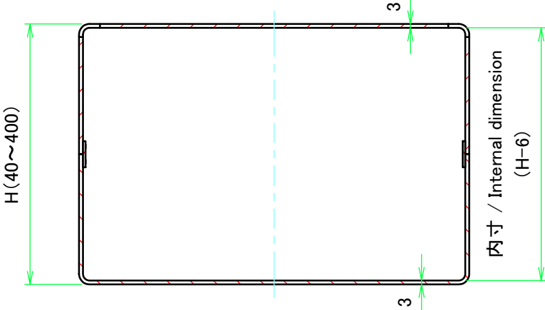
D-D ( 1 : 4 )
