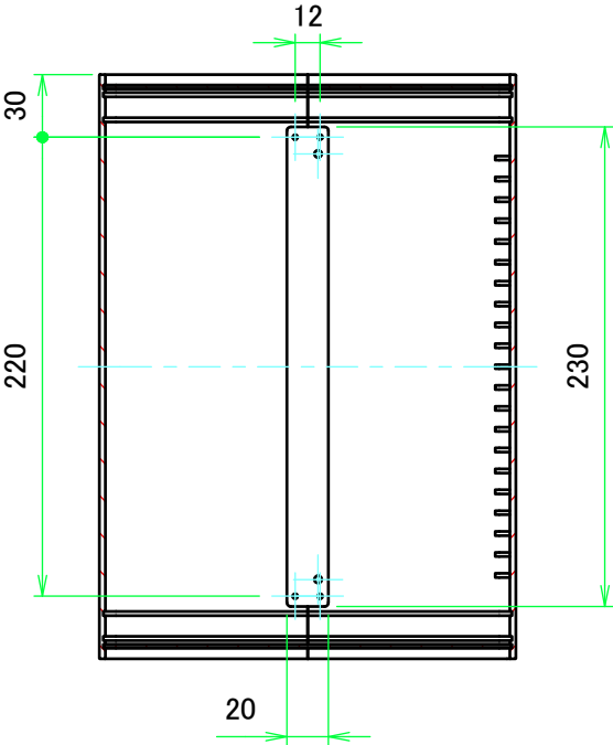
A-A ( 1 : 4 )
