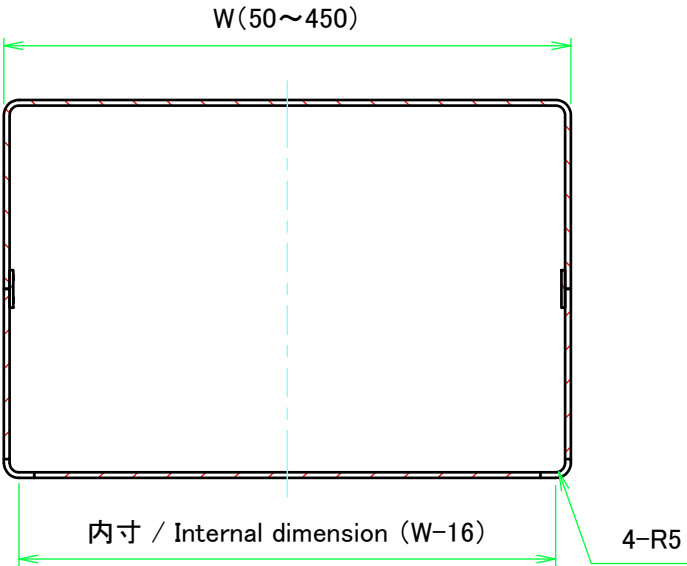
C-C ( 1 : 4 )
