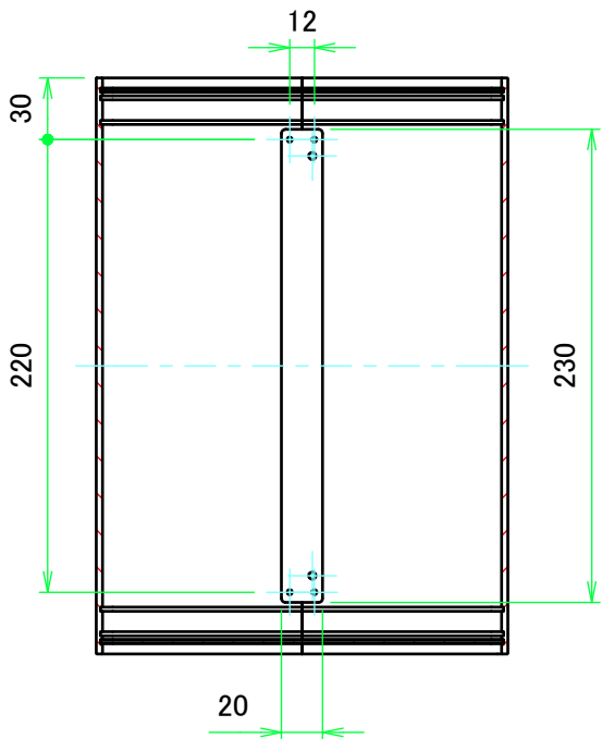
A-A ( 1 : 4 )
