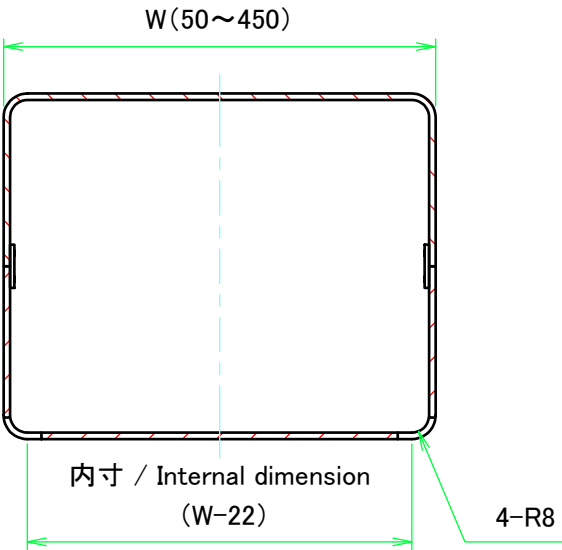
C-C ( 1 : 3.5 )
