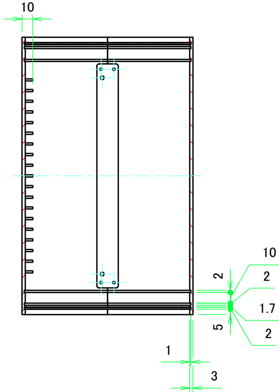
B-B ( 1 : 3.5 )
