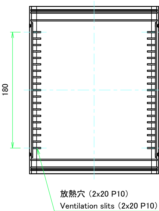
上カバー(内視) Top cover (Internal view)
