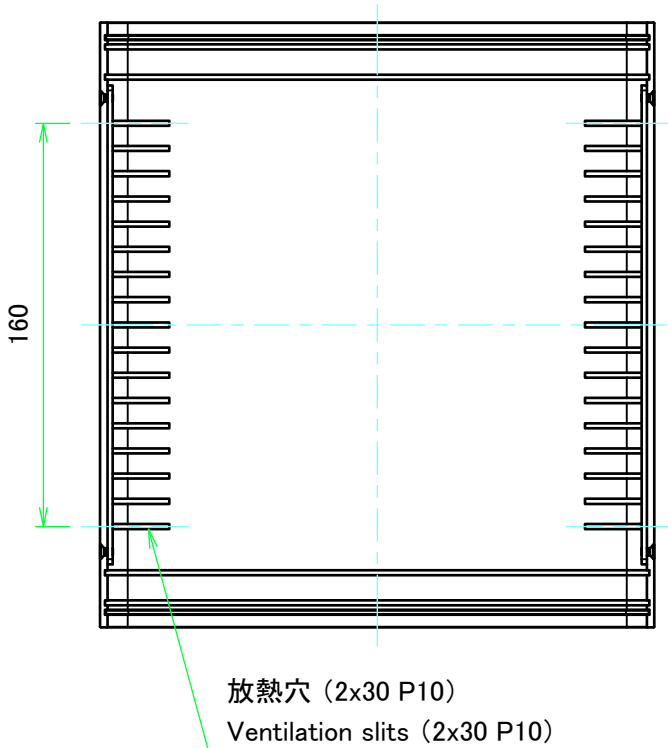
上カバー(内視) Top cover (Internal view)
