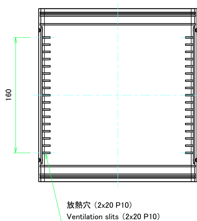
上カバー(内視) Top cover (Internal view)
