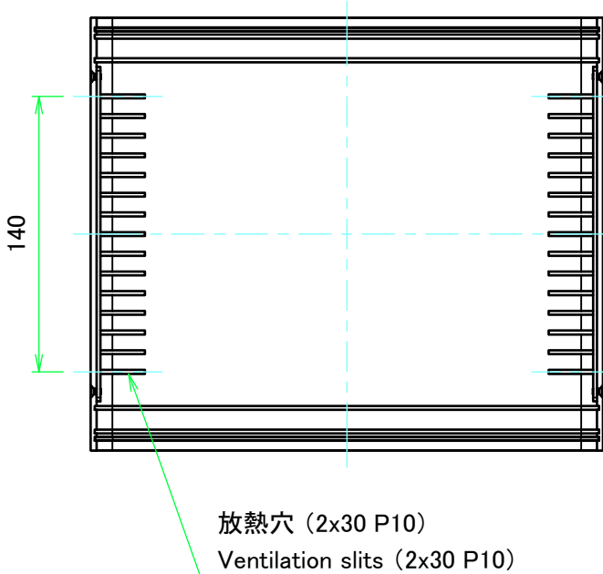
上カバー(内視) Top cover (Internal view)
