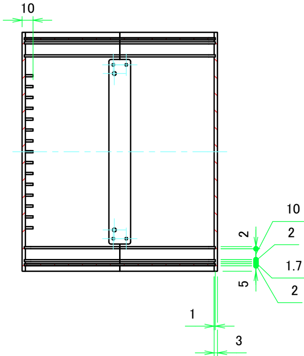
B-B ( 1 : 3.5 )
