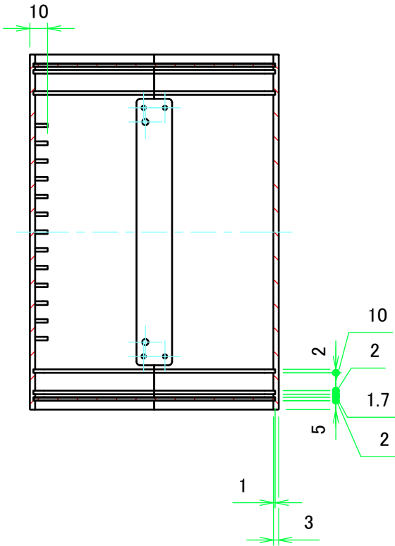
B-B ( 1 : 3 )
