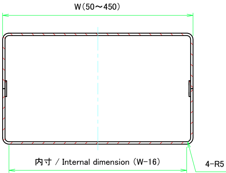
C-C ( 1 : 3 )
