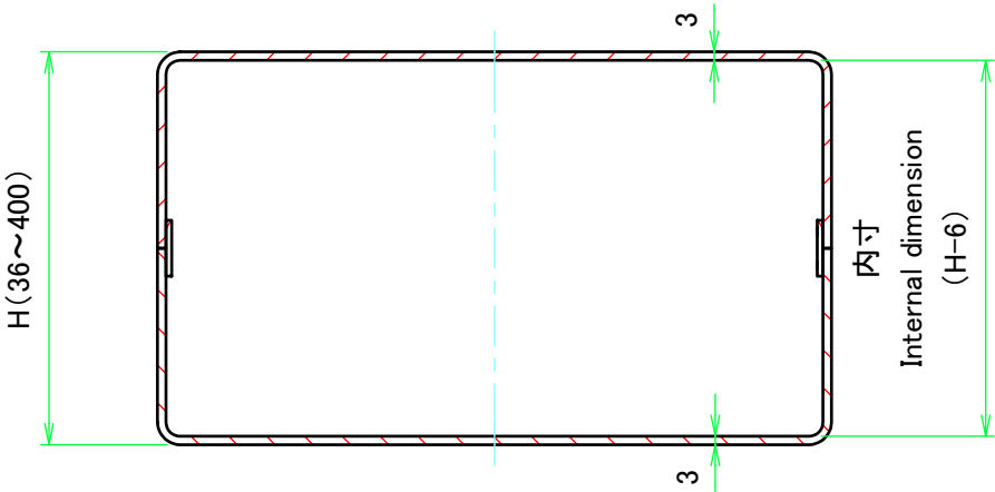
D-D ( 1 : 3 )
