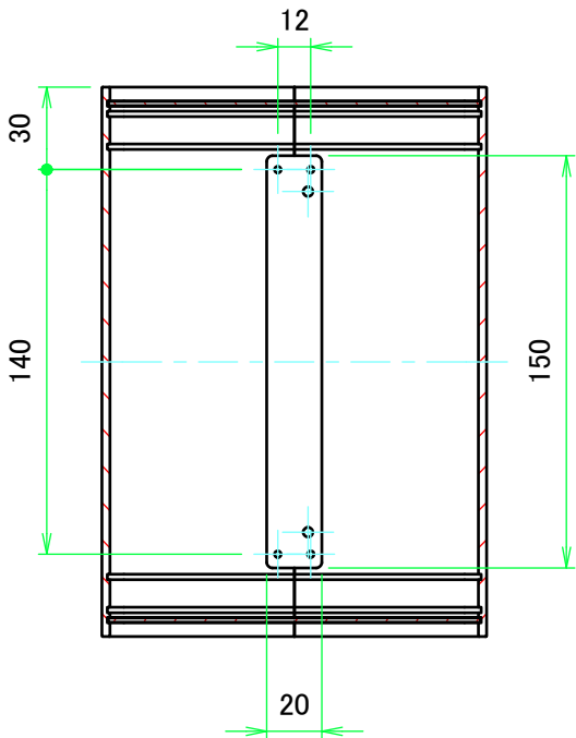
A-A ( 1 : 3 )
