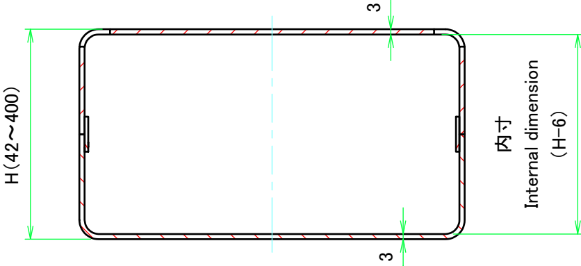
D-D (1:3)
