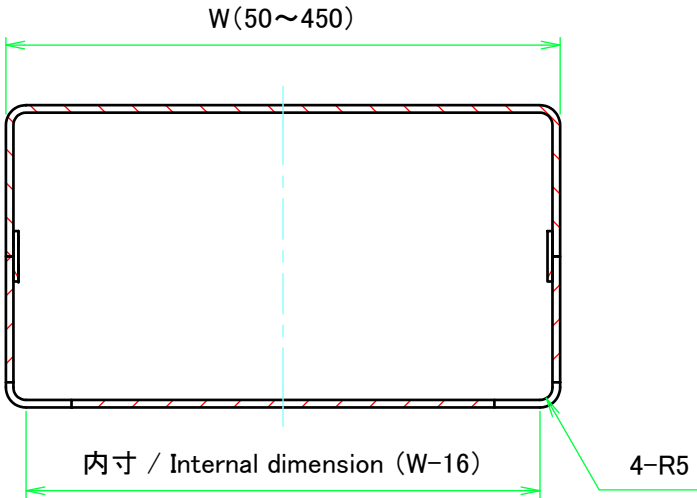
C-C ( 1 : 3 )
