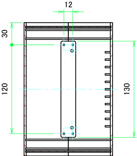
A-A ( 1 : 3 )
