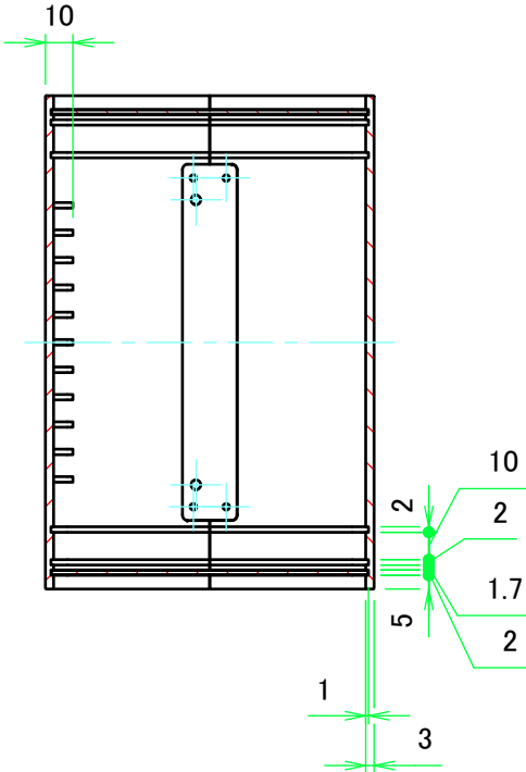
B-B ( 1 : 3 )
