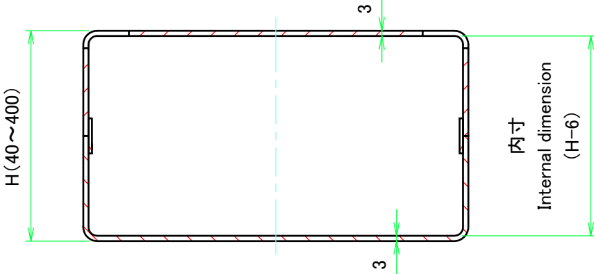
D-D ( 1 : 3 )
