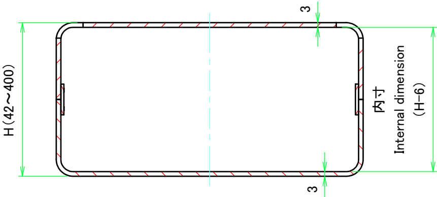
D-D ( 1 : 2.5 )
