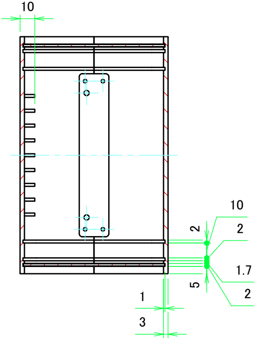
B-B ( 1 : 2.5 )
