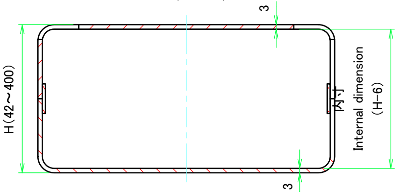
D-D ( 1 : 2.5 )
