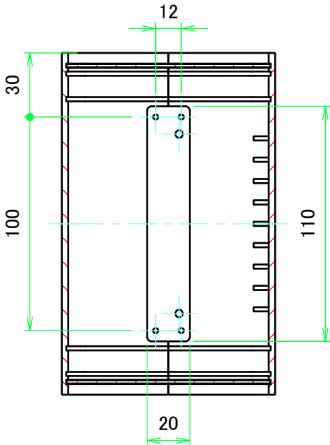
A-A ( 1 : 2.5 )
