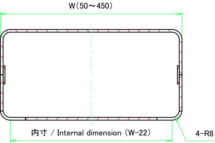
C-C ( 1 : 2.5 )
