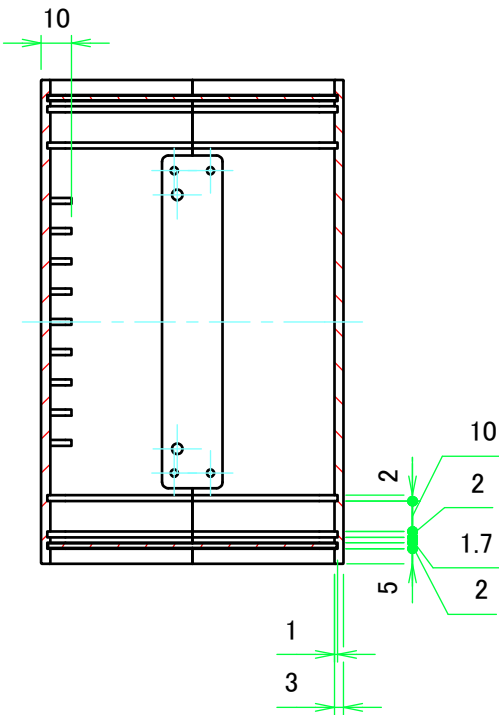
B-B ( 1 : 2.5 )
