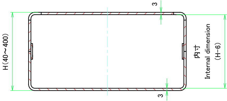
D-D ( 1 : 2.5 )
