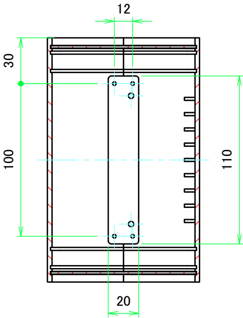
A-A ( 1 : 2.5 )
