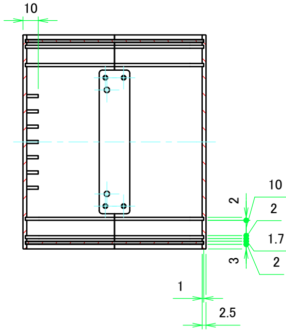
B-B ( 1 : 2.5 )
