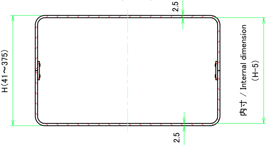
D-D ( 1 : 2.5 )
