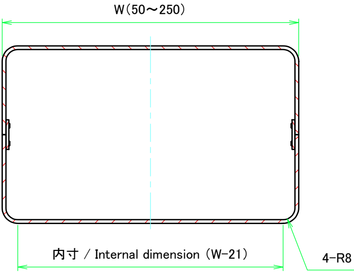
C-C ( 1 : 2.5 )
