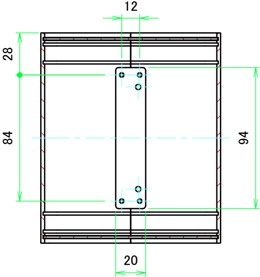
A-A ( 1 : 2.5 )
