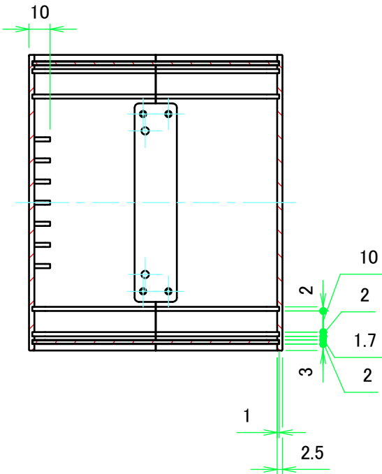
B-B ( 1 : 2.5 )
