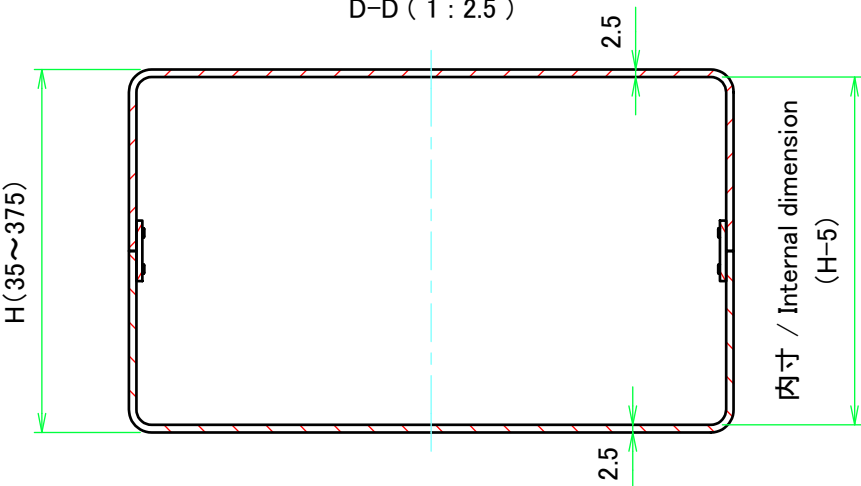
D-D ( 1 : 2.5 )
