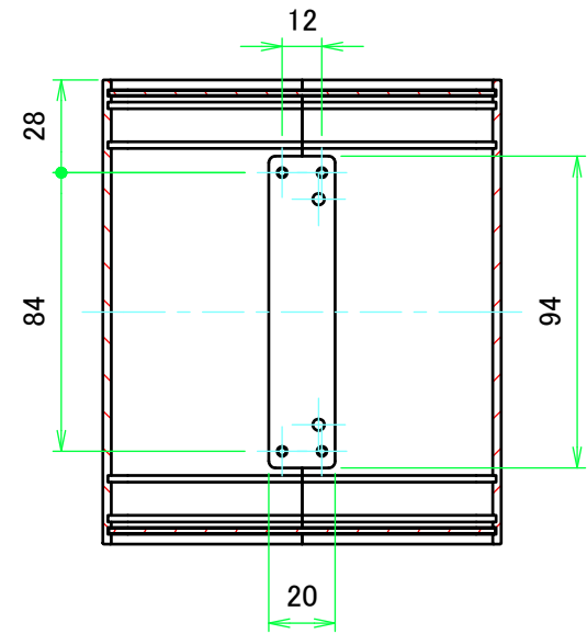
A-A ( 1 : 2.5 )
