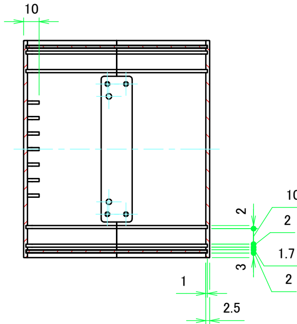
B-B ( 1 : 2.5 )
