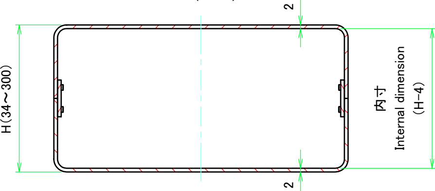
D-D ( 1 : 2 )
